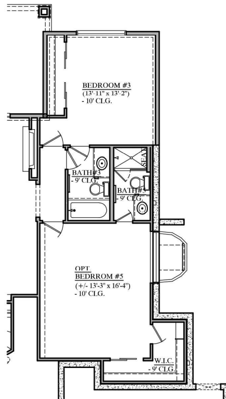
OPTIONAL BEDROOM #5
